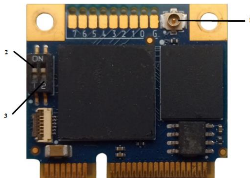
Рис. 2. Расположение основных элементов «КТ-521»
