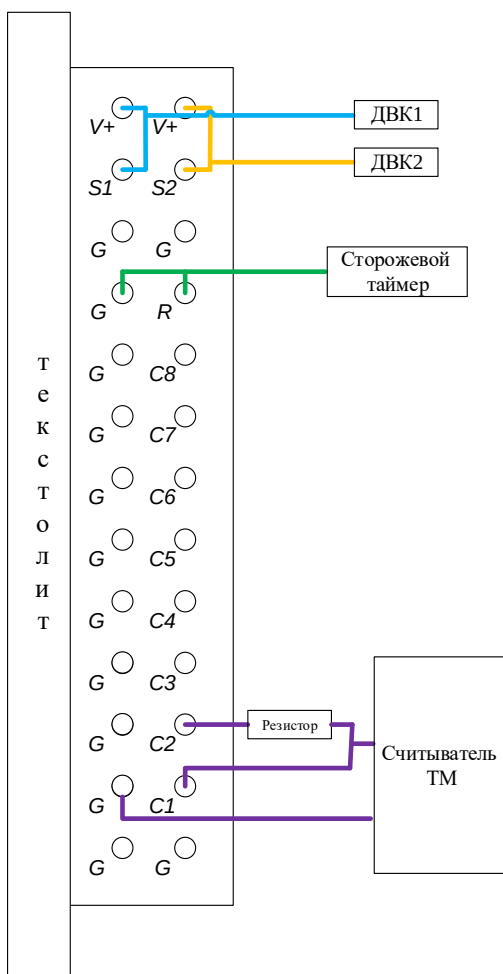
Рис. 4. Схема подключения ДВК, сторожевого таймера и считывателя Touch Memory к штыревым разъемам на плате «КТ-500»
