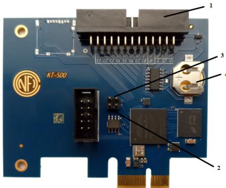
Рис. 1. Расположение основных элементов «КТ-500»
