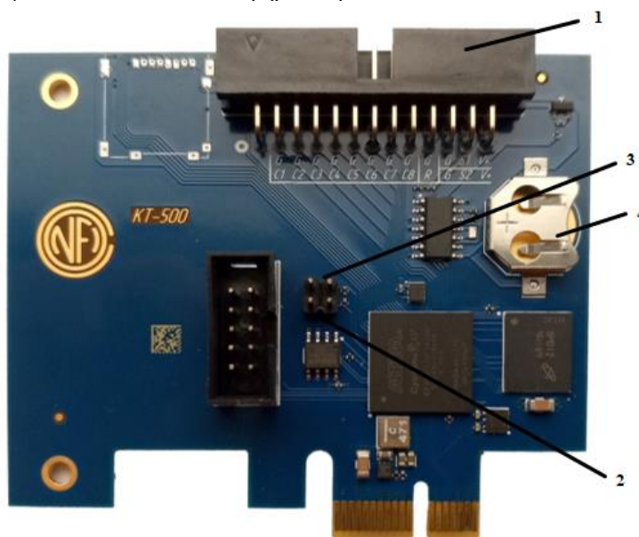
Рис. 1. Плата «КТ-500» и расположение ее основных элементов
