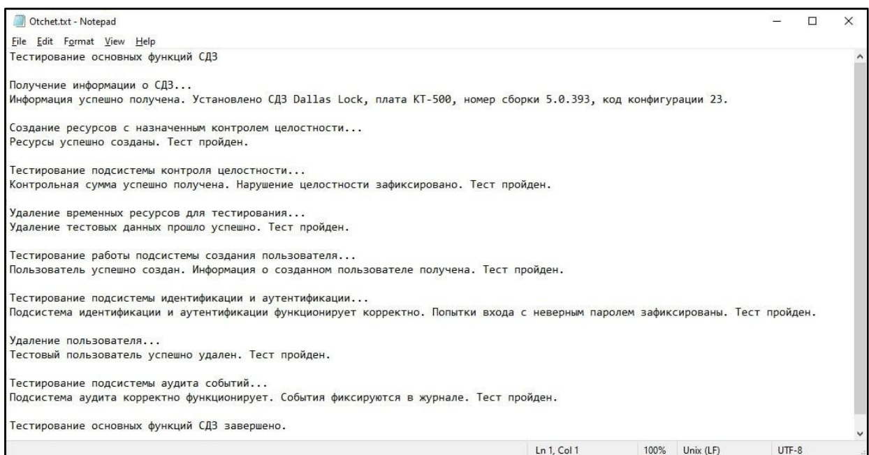
Рис. 67. Сохраненный отчет
