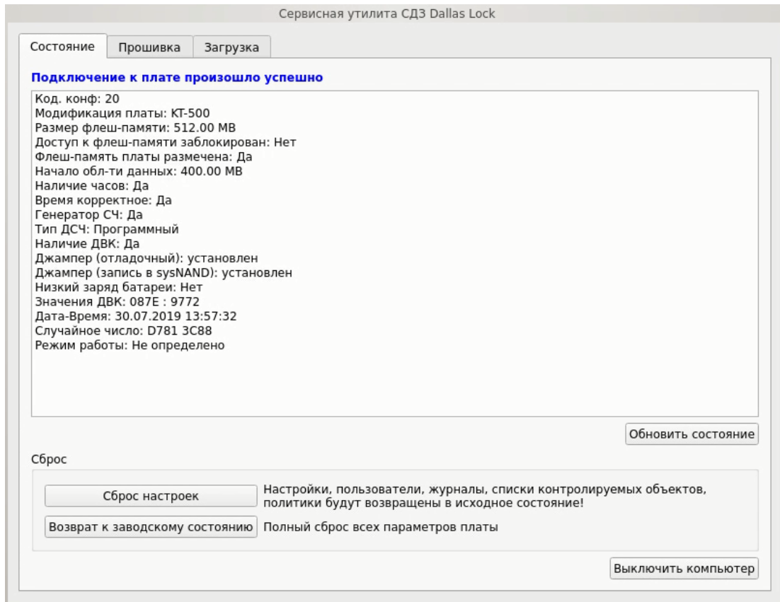
Рис. 69. Сервисная утилита
