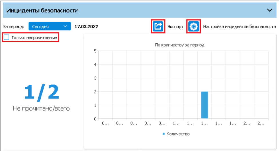
Рис. 46. Настройка инцидентов безопасности
