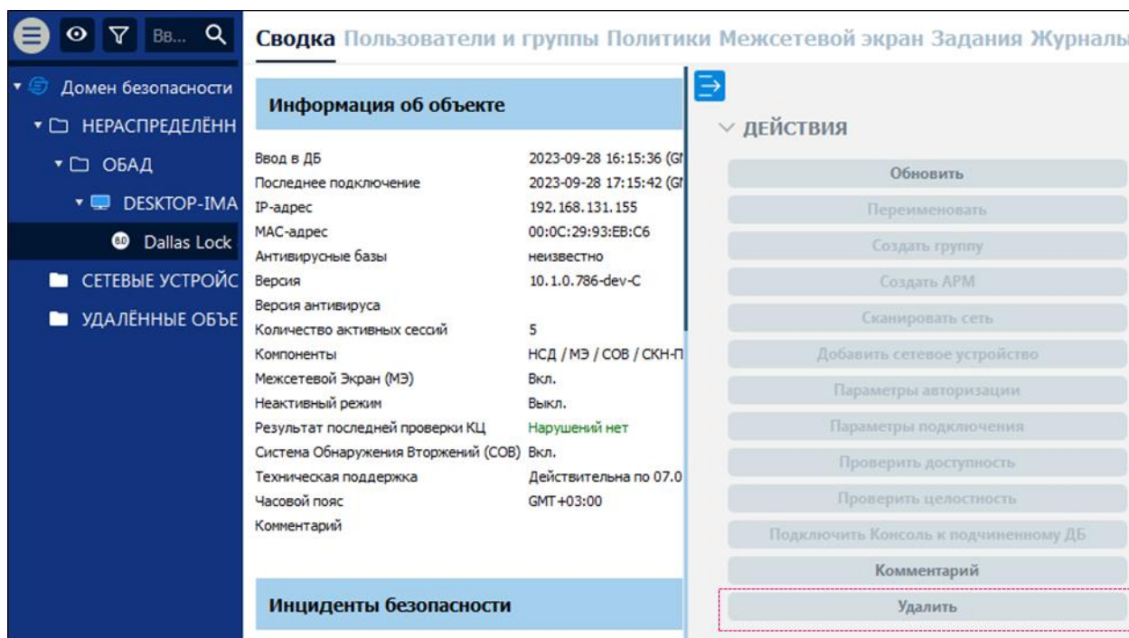
Рис. 115. Удаление посредством панели «Действия»
