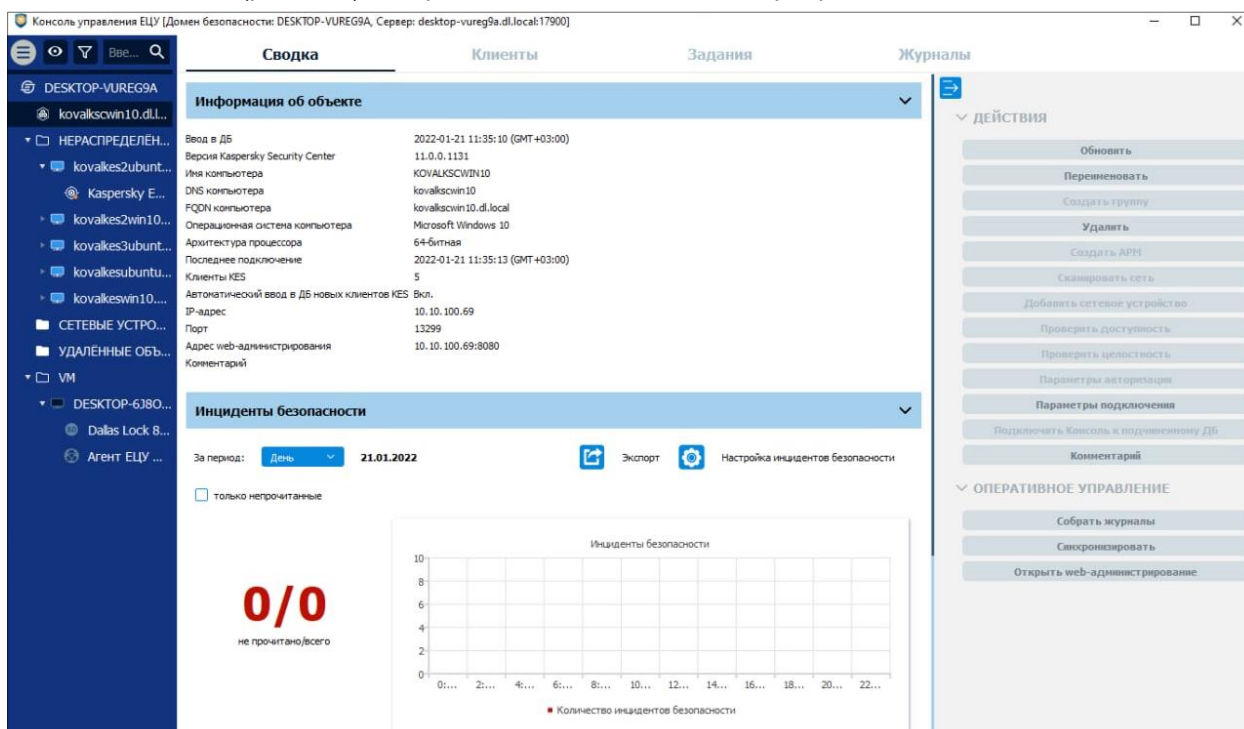
Рис. 245. Вкладка «Сводка» Kaspersky Security Center
