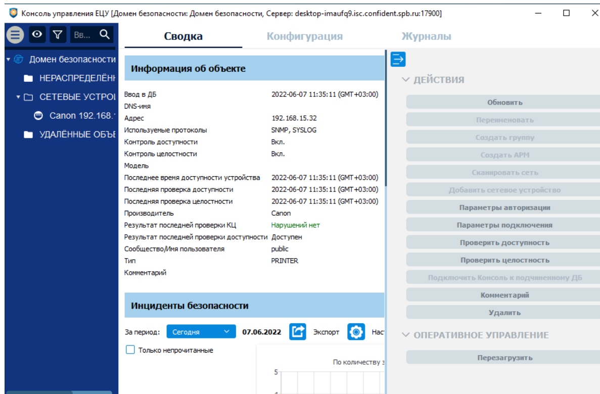
Рис. 262. Сводка сетевого устройства
