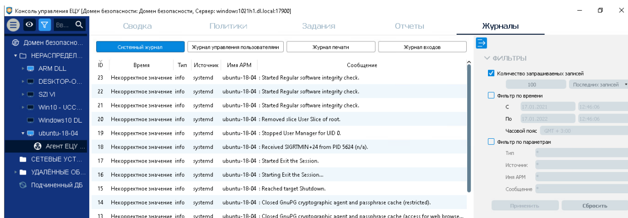
Рис. 238. Журналы Агента ЕЦУ Linux
