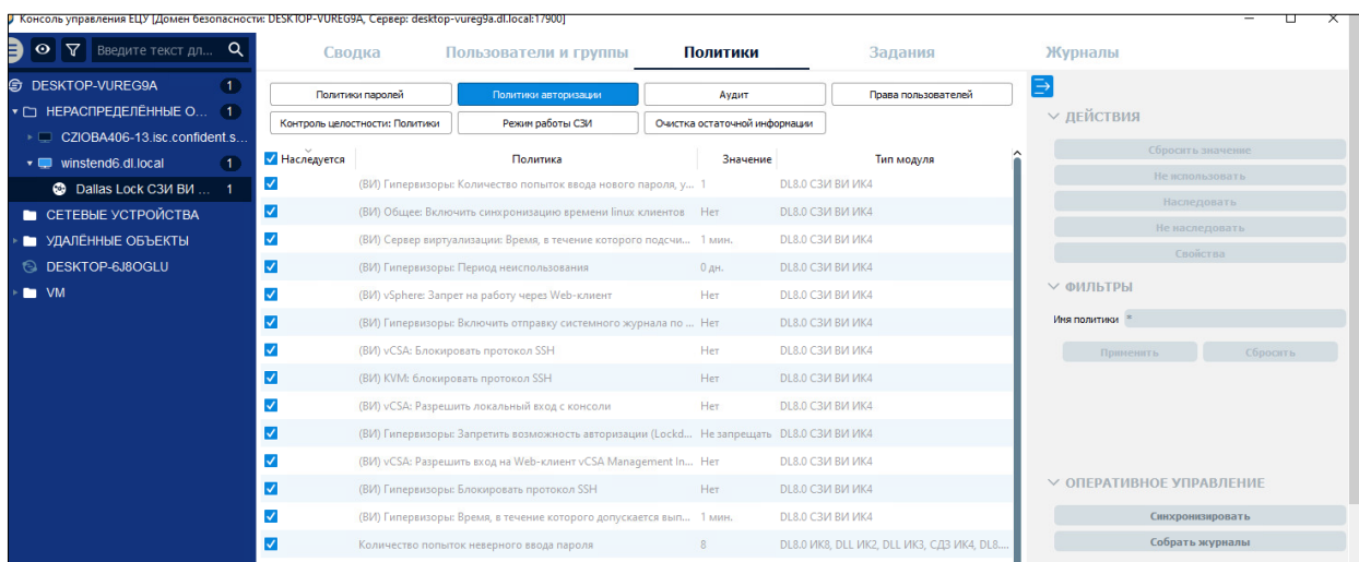
Рис. 190. Политики модуля Dallas Lock C3I BI
