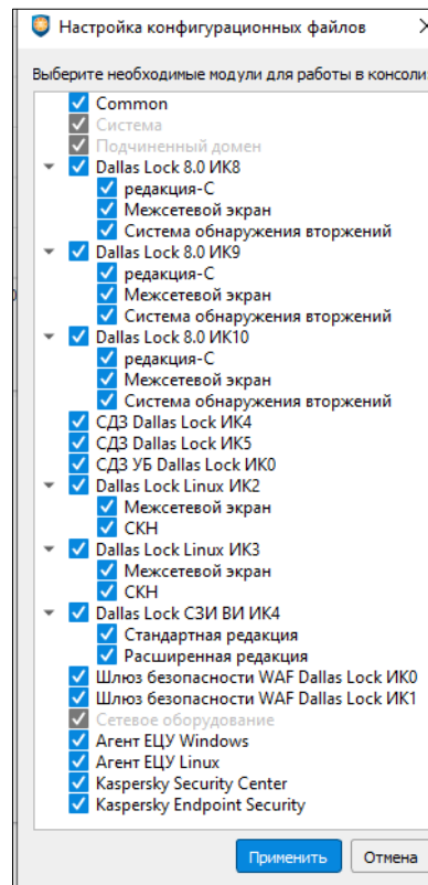
Рис. 57. Настройка конфигурационных файлов
