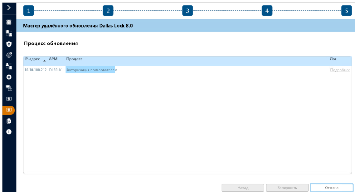
Рис. 236. Процесс обновления
