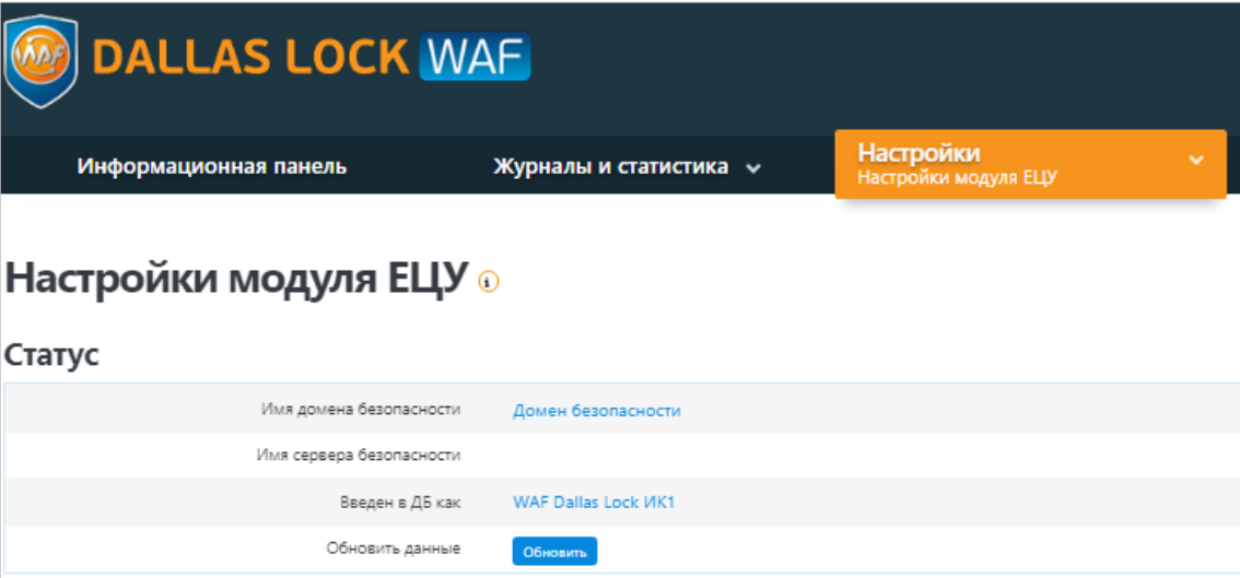
Рис. 289. Кнопка «Обновить»
