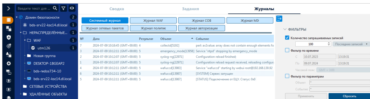
Рис. 292. Вкладка «Журналы»
