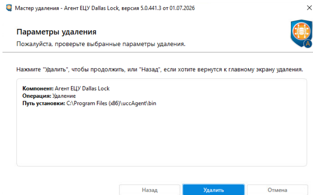
Рис. 311. Параметры удаления
