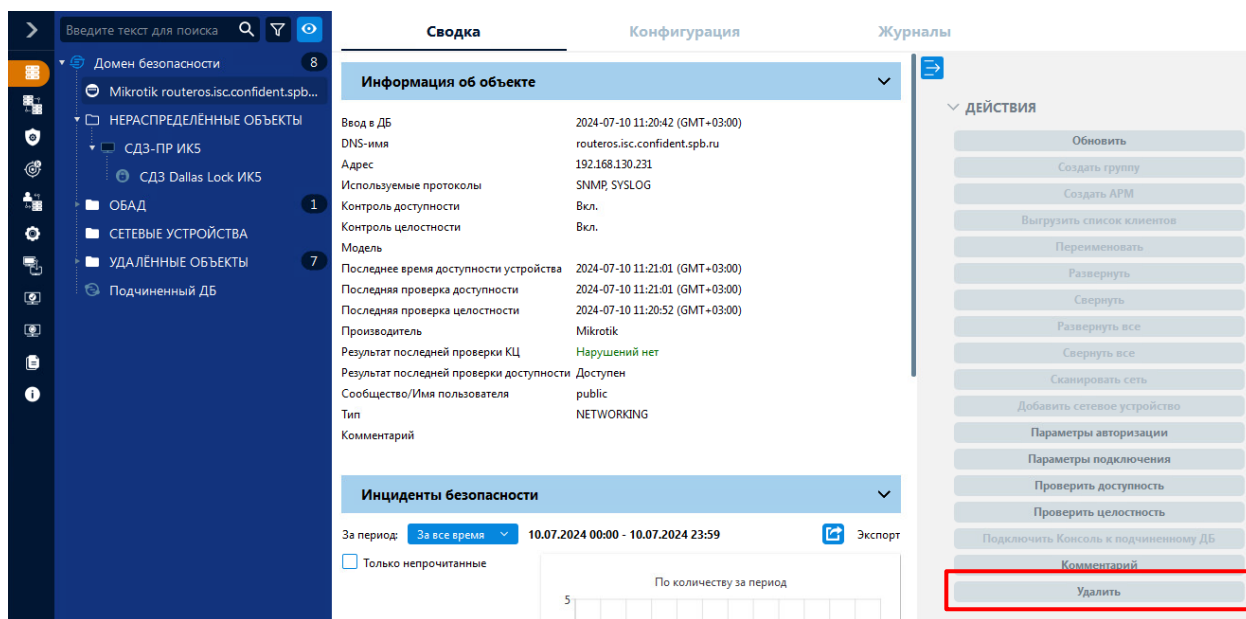
Рис. 351. Удаление посредством панели «Действия»
