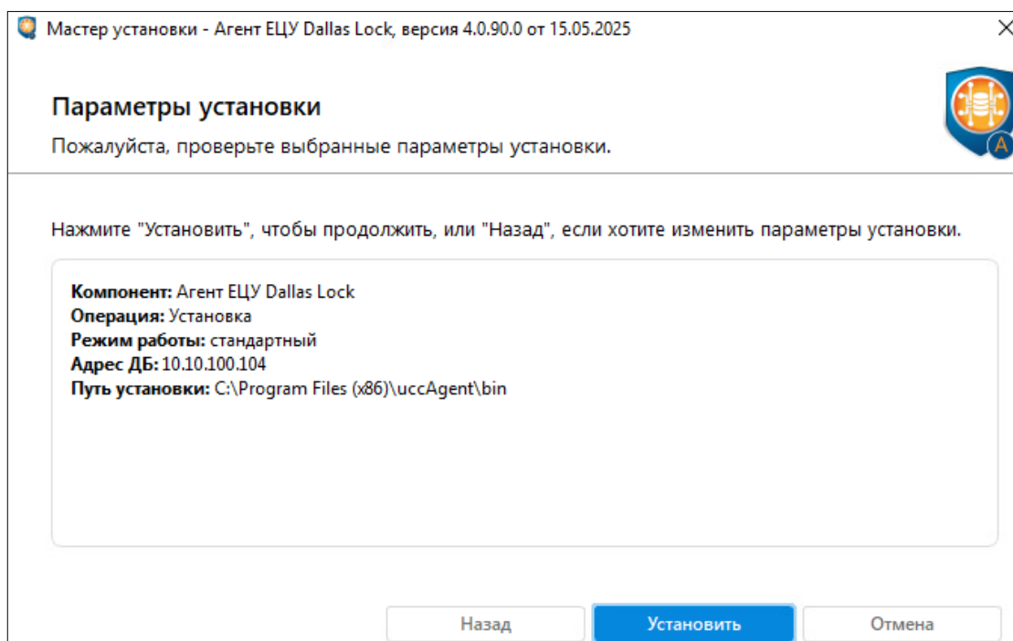
Рис. 299. Проверка параметров установки Агента ЕЦУ
