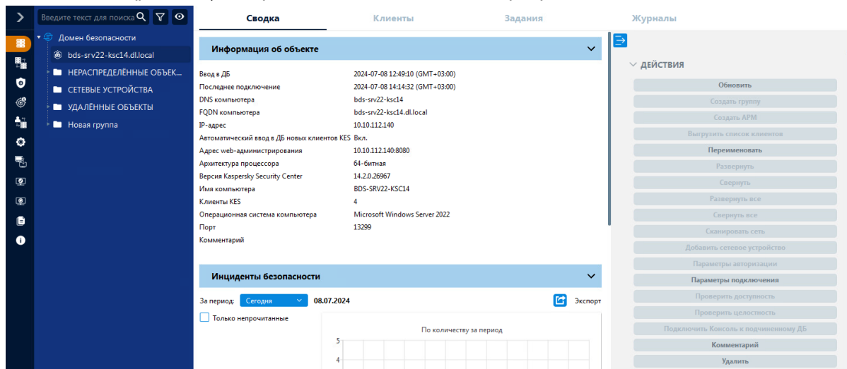
Рис. 334. Вкладка «Сводка» Kaspersky Security Center
