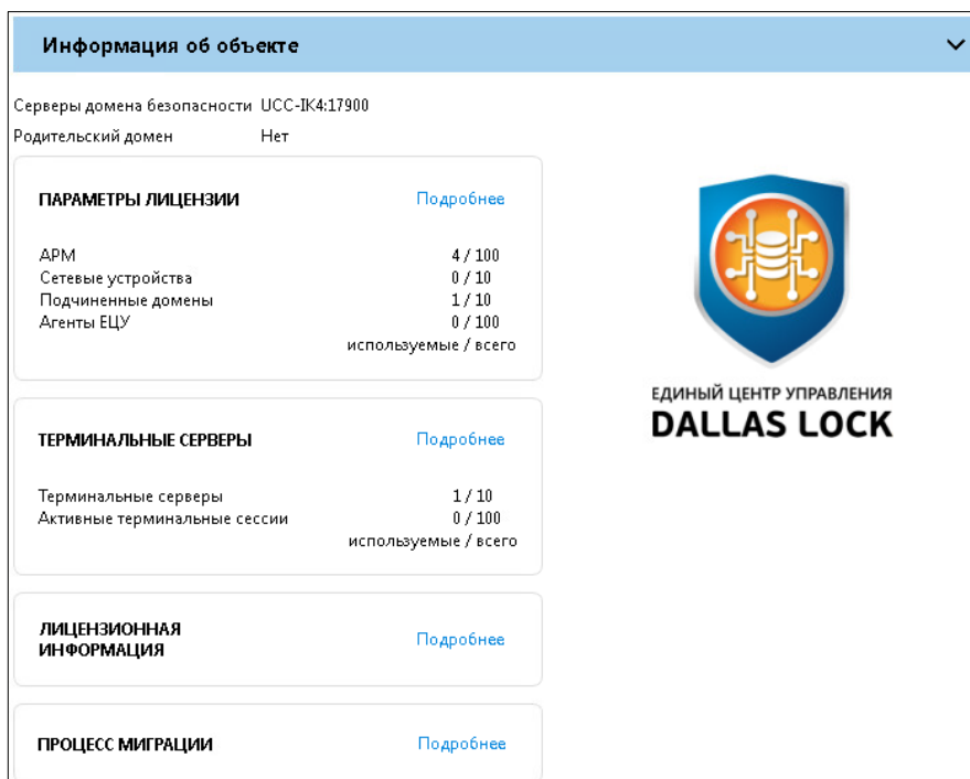
Рис. 74. Раздел «Информация об объекте»
